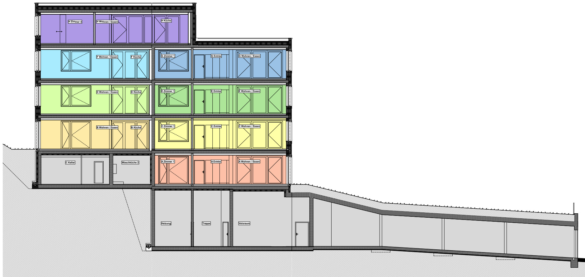
Schnitt A-A
