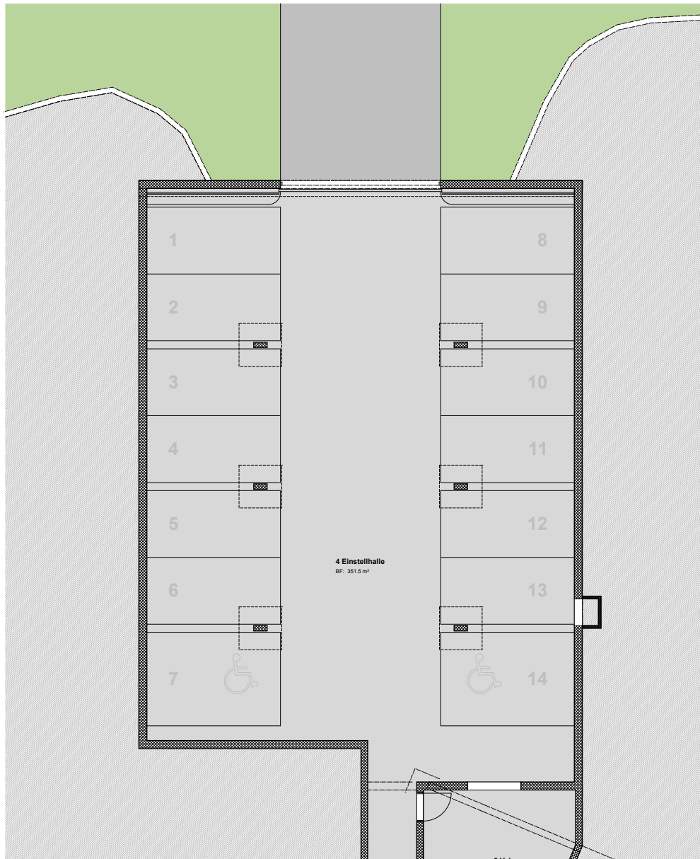
Einstellhalle
