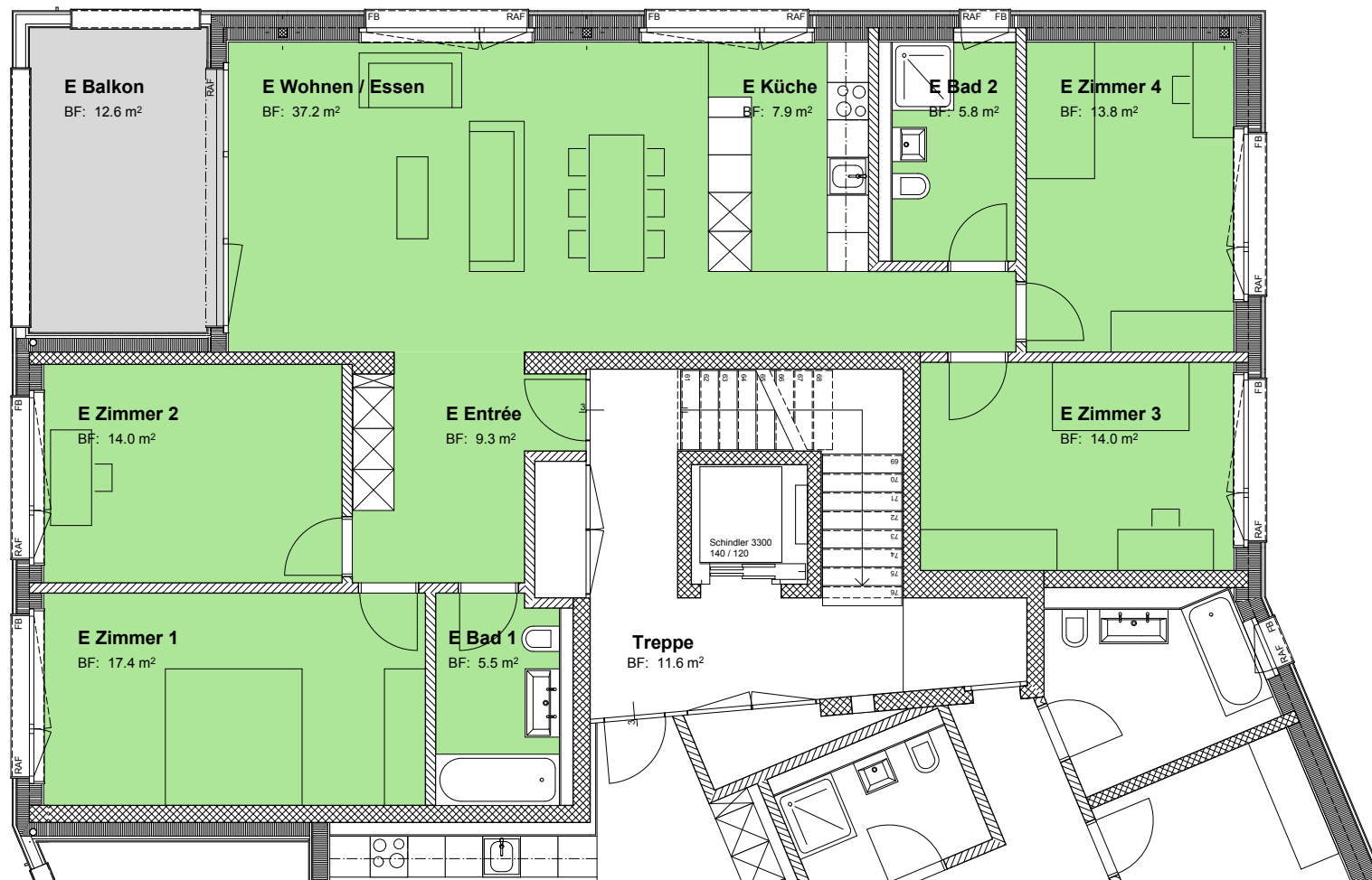
1. Obergeschoss E Wohnung Nord 5½ Zimmer 124.9 m 2
